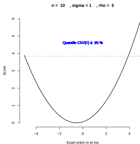
FIGURE 10 – Influence d'une très faible taille d'échantillon.
