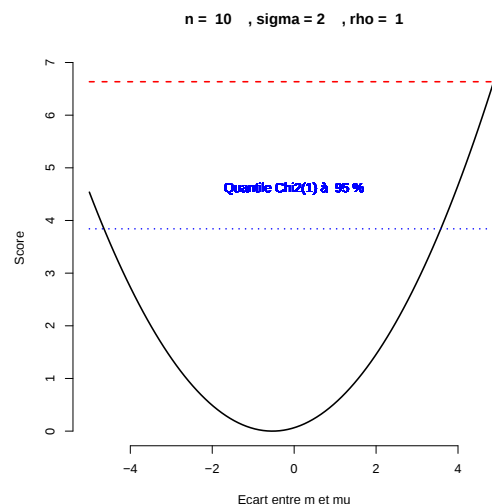
FIGURE 9 – Influence d'un \sigma plus large.
