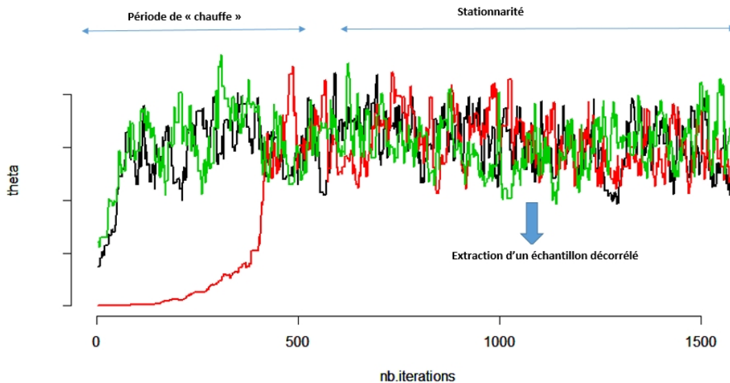
FIGURE 18 – Trois chaînes MCMC convergeant en parallèle vers la même loi-cible a posteriori . La période de chauffe correspond au nombre d'itérations nécessaire au mélange des chaînes, qui est un indicateur de l'atteinte de la stationnarité.
