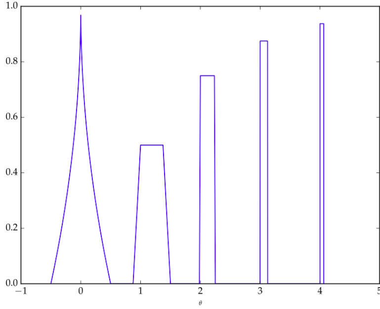
FIGURE 1 – Exemple d’une loi a posteriori dont le MAP n’est pas la limite d’une suite d’estimateurs bayésiens. Source : [3].
