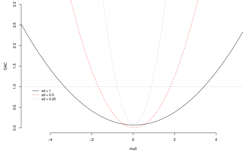
FIGURE 13 – Exemple 6.5.1. Vraie valeur \theta_0 = 0 , taille n = 5
