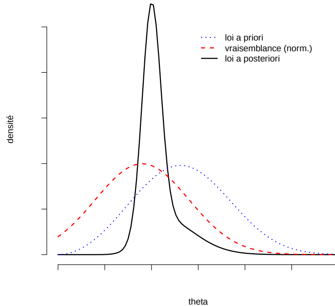
FIGURE 3 – Illustration par les densités du renforcement de l’information sur \theta à partir de la loi a priori et la vraisemblance des données (vue comme fonction de \theta et ici renormalisée).
