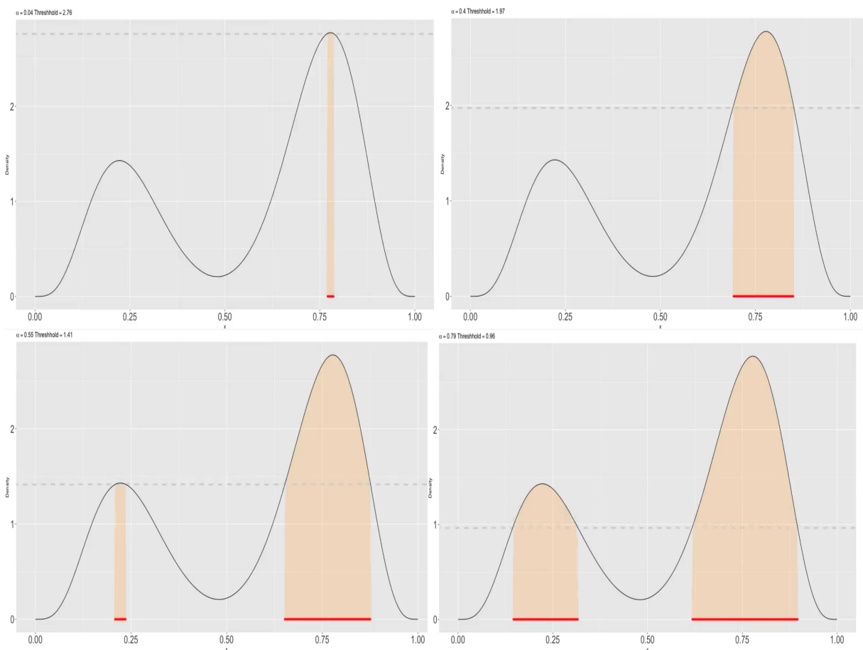
FIGURE 2 – Exemples de régions HPD dans un cas de posterior multimodal, pour un seuil \alpha de 0.04 (en haut à gauche), de 0.4 (en haut à droite), de 0.55 (en bas à gauche) et de 0.79. On perçoit bien que la région HPD n'est pas forcément connexe, comme le serait un intervalle de crédibilité . Crédit : M. Ribatet
